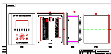
JSH-200外形及开孔图
