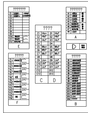
JSH-3108 主变接地装置有载调压端子图
