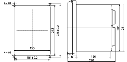
JSH-300系列保护测控装置屏柜开孔图
