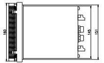
JSH-300系列保护测控装置屏柜开孔图
